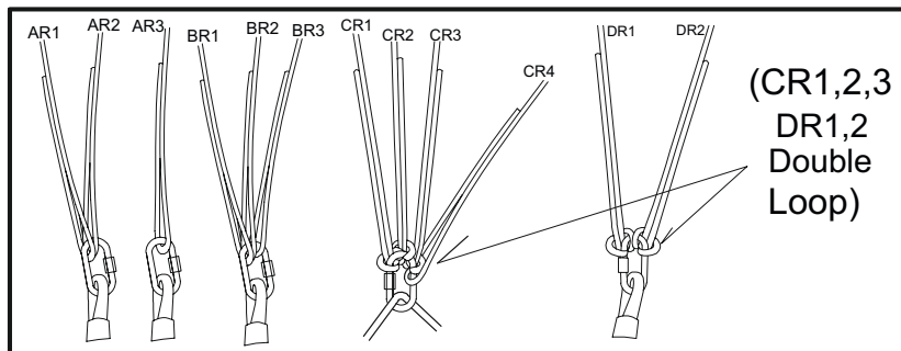
Werksauslieferung mit doppeltem Loop der C und D-Stammleinen für die Trimmung bei Alterung
